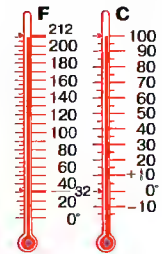
Градус Фаренгейта Порівняння шкал Фаренгейта і Цельсія (температури замерзання та кипіння води позначено малими стрілками)
